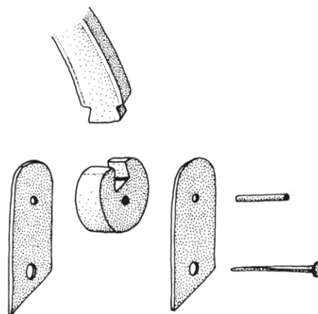
Fig. 4 : Construction de l'anse avec son attache, vue éclatée en perspective.
