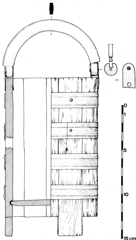
Fig. 5 : Nécropole de Roanne, reconstitution du seau ; éch. 1/2.
